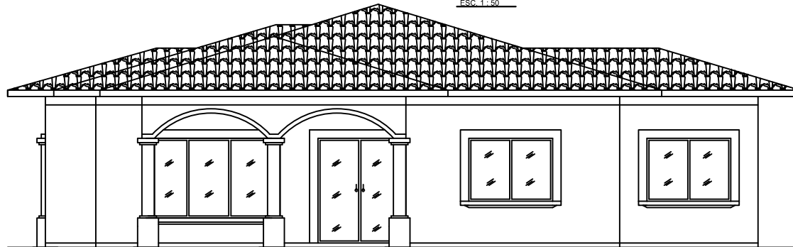
ELEVACION POSTERIOR
